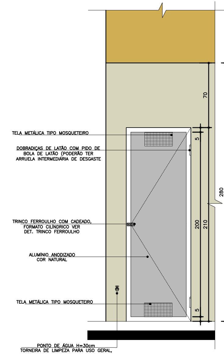
08 Elevação 02 ABRIGO DE RESÍDUOS COMUNS Esc.: 1:25
