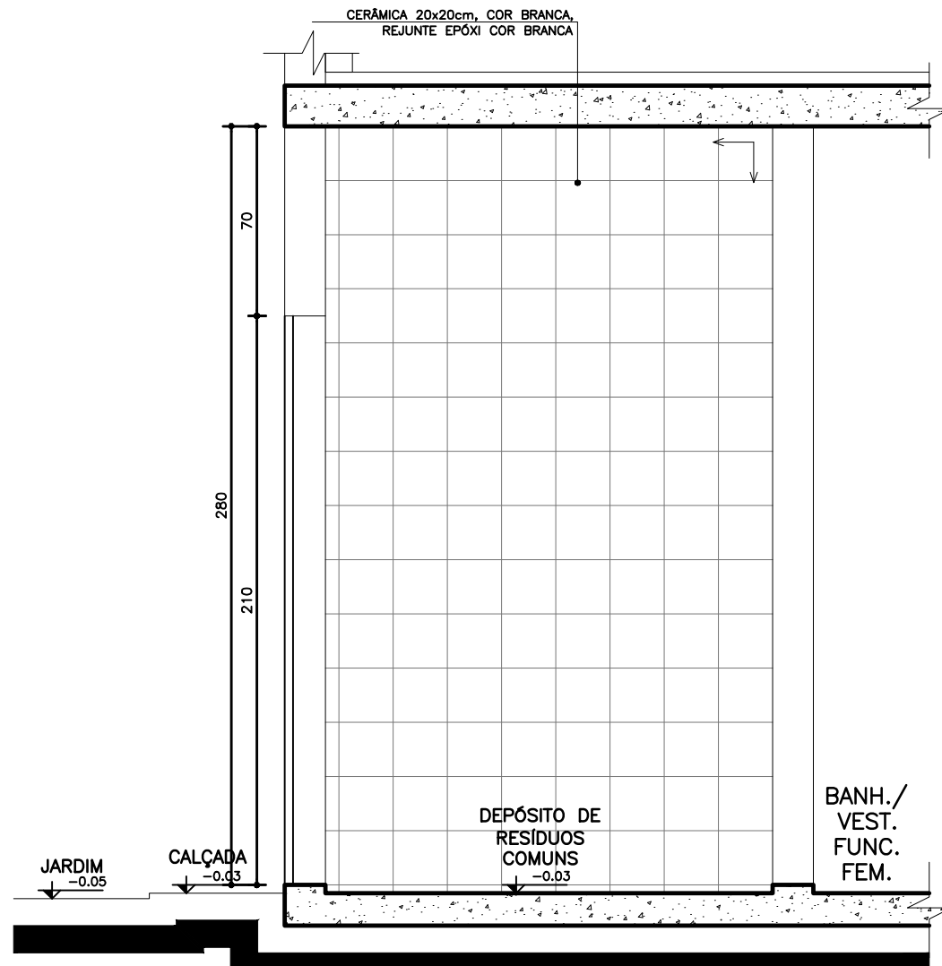
06 Seção AA' ABRIGO DE RESÍDUOS COMUNS Esc.: 1:25
